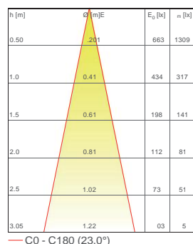
— C0 - C180 (23,0°)
