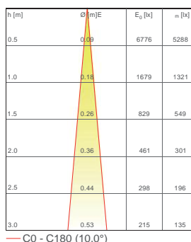
— C0 - C180 (10,0°)
