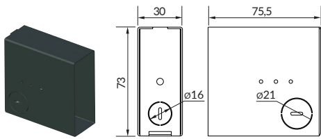
Boîtier d'encastrement Art. Nr. HB.004
