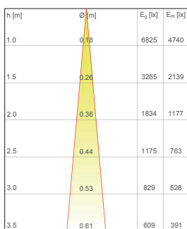
— C0 - C180 (10,0°)
